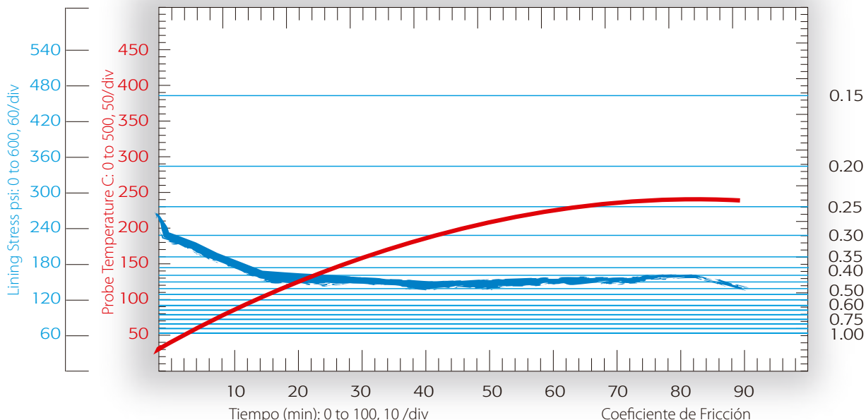
Gráfico FAST (Comportamiento del Coeficiente de Fricción):
